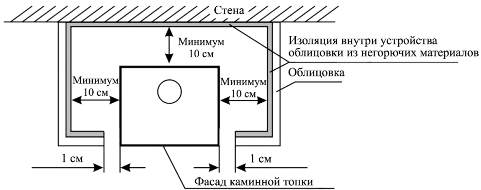
Рис. 3. Вид сверху
