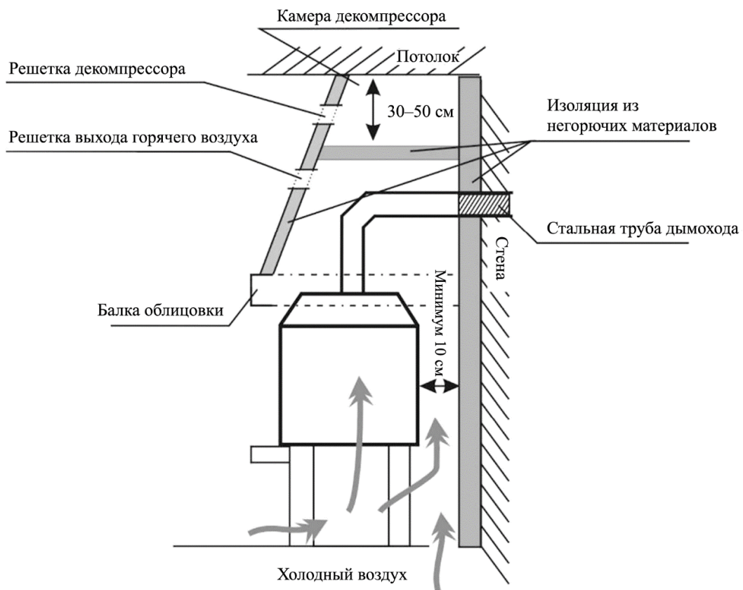
Рис. 4. Вид сбоку
