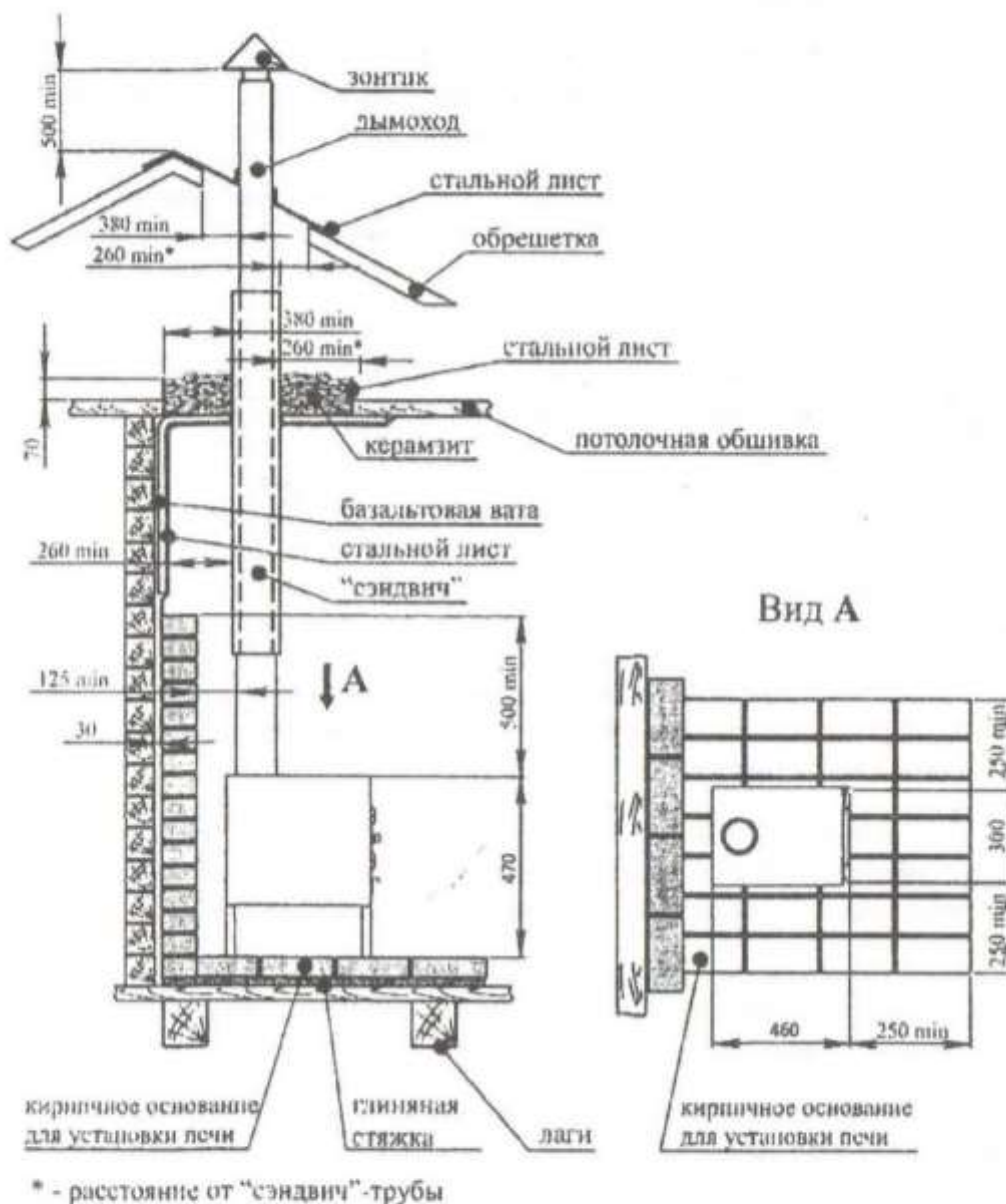
Рис. Схема установки печи
